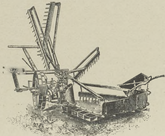
102-ik ábra. Marokrakó aratógép gyommaggyűjtő fiókkal.
