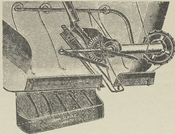
103-ik ábra. Magfogó egy kéveköti aratógéphez.
