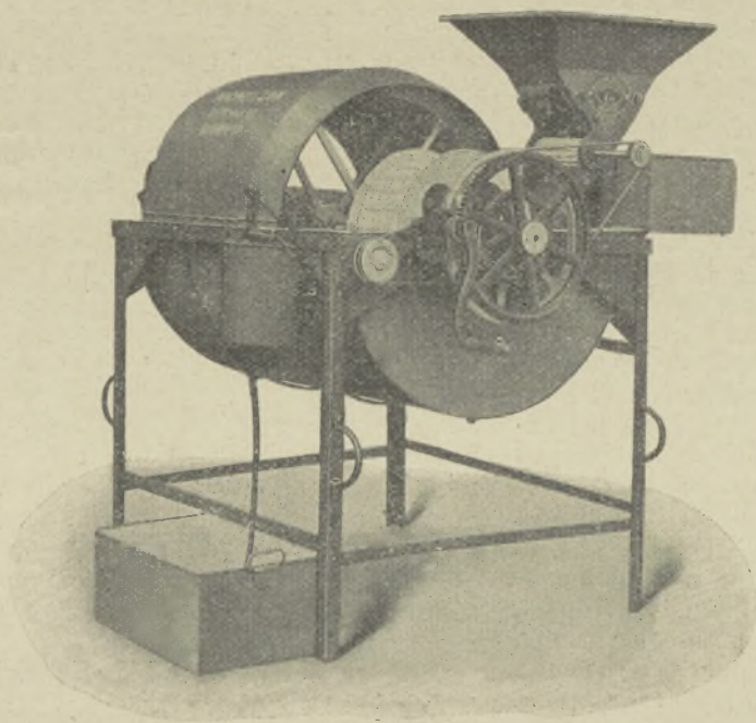
52-ik ábra. A Huszár-féle gabonacsávázó-gép kétoldalról nézve.
