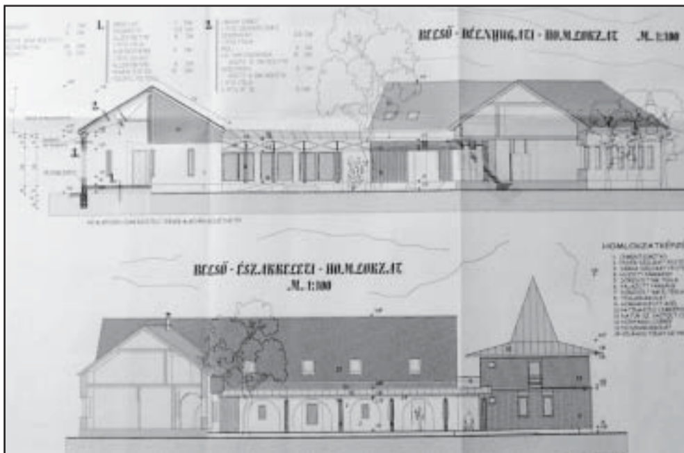
A belső rész délnyugati és északkeleti homlokzatának rajza
