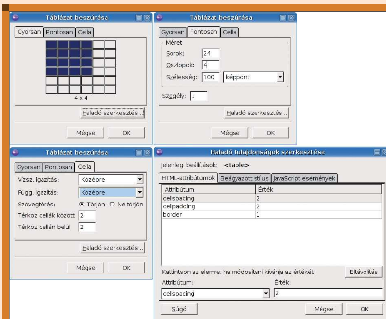
■ 4. ábra Táblázat beállításai
