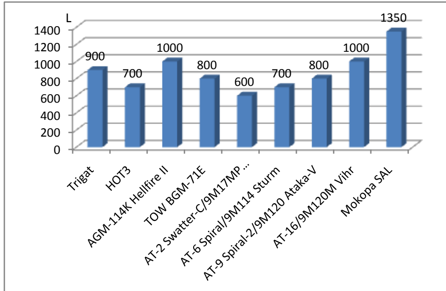
3. ábra. A helikopterfedélzeti irányítható páncéltörő rakéták maximális páncélatütőképessége
