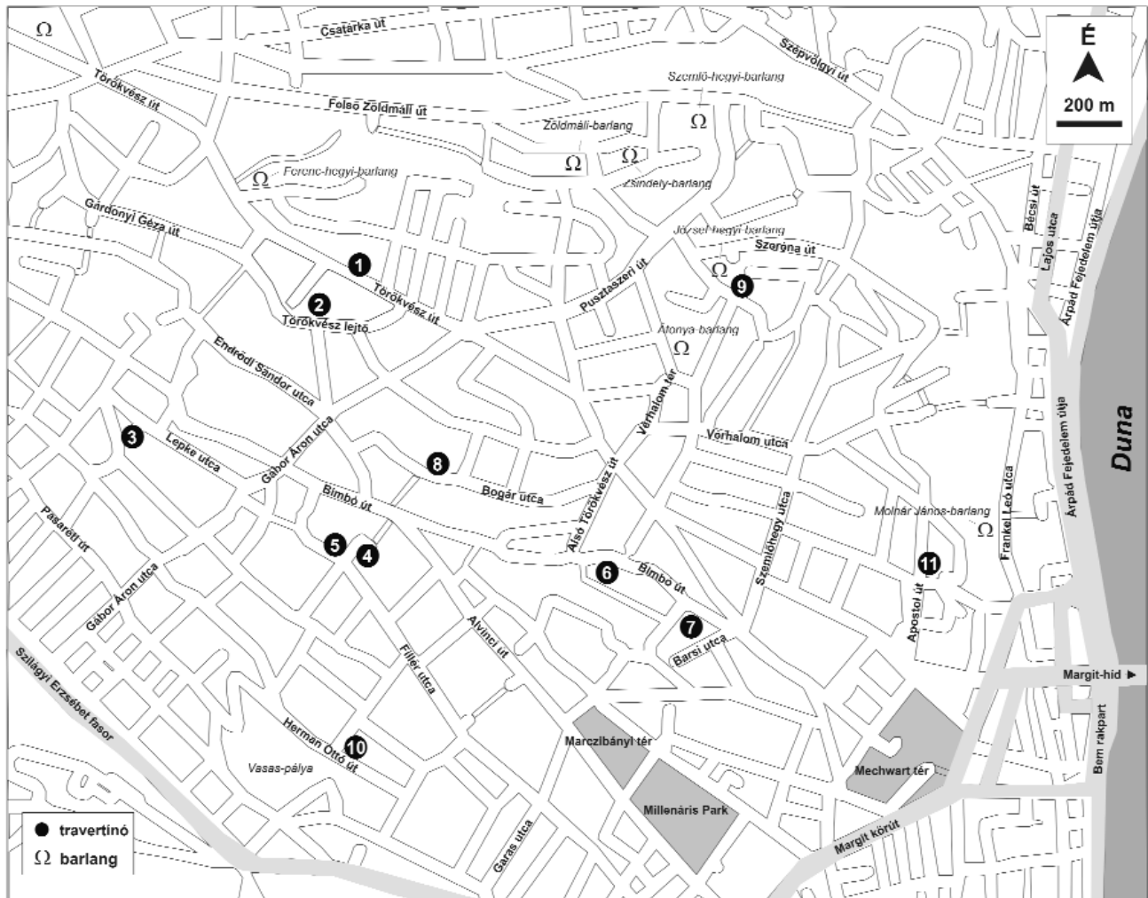
3. ábra. A Rózsadombi édesvízmészke-előfordulások és barlangok elhelyezkedése (a térkép a Google, Tele Atlas internetes utcaterképének módosított változata). A barlangok LEÉL-ÖSSY & SURÁNYI (2003), míg az édesvízi mészkövek KELE (2009) alapján lettek feltüntetve
