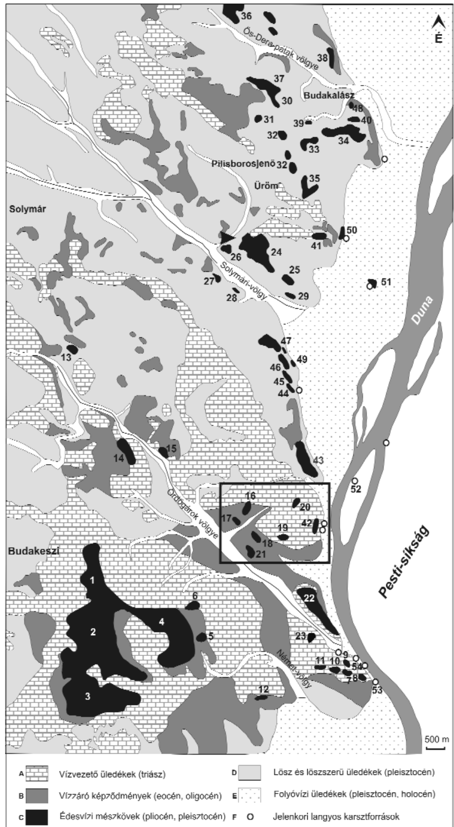
1. ábra. A Budai-hegység vázlatos földtani térképe a jelentősebb édesvízmész-kő-előfordulások feltüntetésével (módosítva SCHEUER & SCHWEITZER 1974, valamint KELE 2009 alapján)
