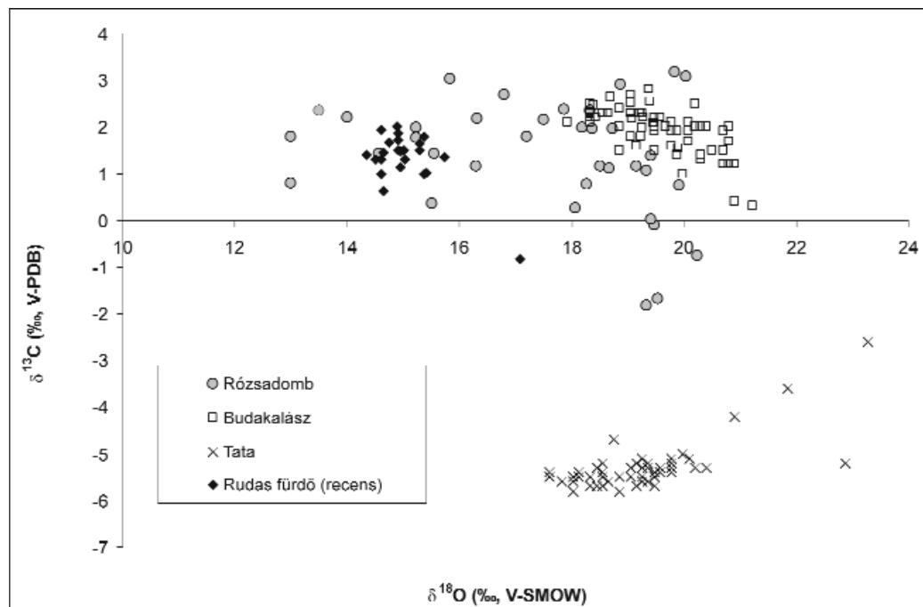
7. ábra. A rózsadombi travertínok stabilizotópos összetételének összevetése a felső-pleisztocén Tata, Porhanyó-bánya (Nyugat-Gerecse, KELE et al. 2006), a pleisztocén Budakalász (Budai-hegység, KELE et al. 2003) travertínóinak már korábban publikált izotópos értékeivel, valamint a Rudas fürdő (Budapest) recens karbonátkiválásának (VERES 2007) izotópos értékeivel
