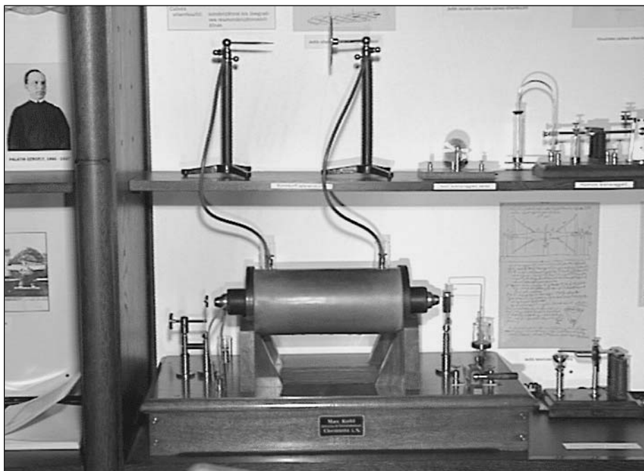
Szikrainduktor
